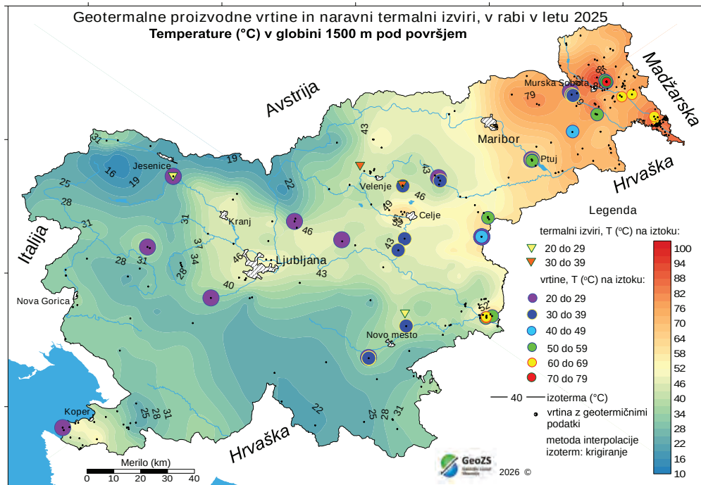
Slika 9: Proizvodne geotermalne vrtine in naravni termalni izviri v uporabi v letu 2025, porazdeljeni glede na poprečno letno temperaturo termalne vode na ustju vrtin in izvirov (stanje: ob koncu 2025). Karta prikazuje pričakovane temperature v globini 1500 m pod površjem.
