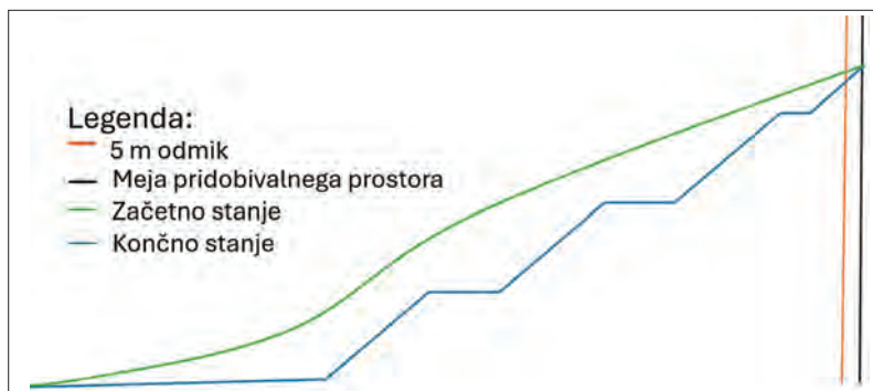
Slika 4: Primer neustreznega načrtovanja – brežina sega v 5 meterski varovalni pas
