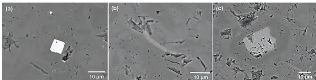
Slika 4: Manj zastopani minerali v dolomitih, opazovani z vrstičnim elektronskim mikroskopom: (a) železov oksid, (b) sljuda in (c) delno raztopljen kalcit
