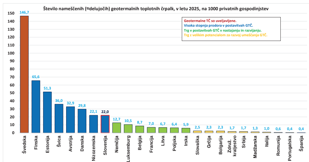
Slika 10: Število nameščenih (≈delujočih) geotermalnih toplotnih črpalk v letu 2025 na 1000 privatnih gospodinjstev v Evropi (EGEC, 2026b); število gospodinjstev po: 2025 Eurostat demographic data; – Podatki za Albanijo, Bosno & Hercegovino, Ciper, Češko, Hrvaško, Latvijo, Malto, Norveško in Sev. Makedonijo v teh raziskavah niso bili na voljo.
