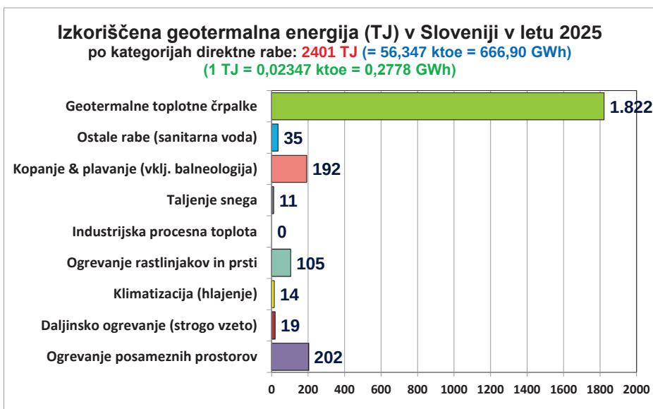
Slika 11: Vsa izkoriščena geotermalna energija v Sloveniji v letu 2025 po kategorijah direktne rabe
