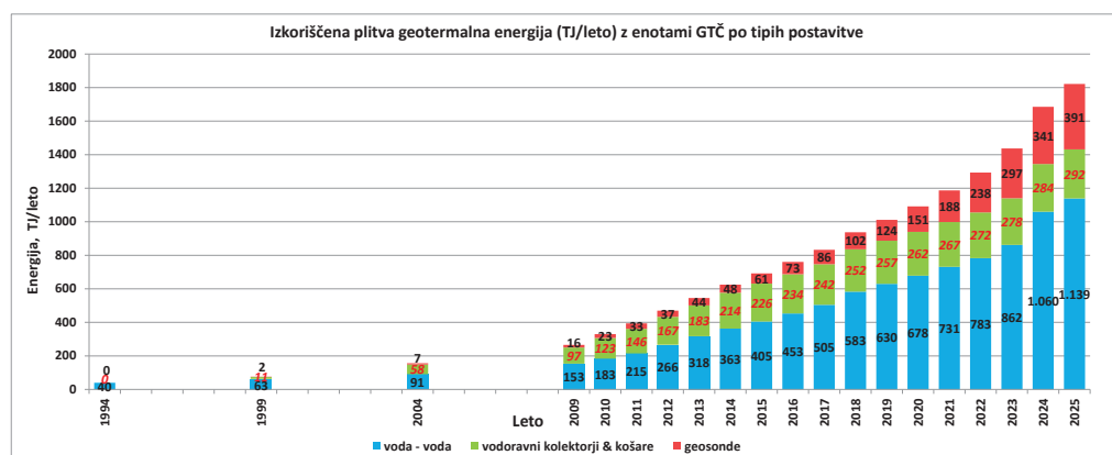
Slika 14: Izkoriščena plitva geotermalna energija z delujočimi enotami GTČ v Sloveniji od začetka vodenja statistike in po vrsti postavitve; skupna izkoriščena plitva GTE v letu 2025: 1821,9 TJ; za leta 1995–2013 so podatki o izkoriščeni energiji po vrsti postavitve le približni.
