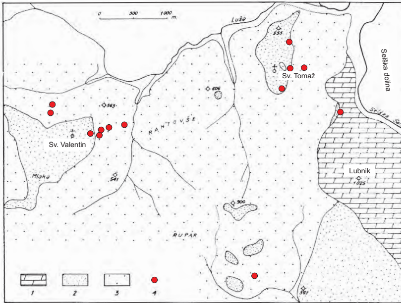
Slika 11: Sveti Tomaž in Sveti Valentin z anomalijami radioaktivnosti. Litologija (legenda spodaj levo): 1 – dolomit in apnenec (srednji trias); 2 – grödenske plasti (srednji perm); 3 – peščenjak, konglomerat in glinasti skrilavec (karbon); 4 – anomalija radioaktivnosti (prirejeno po Omaljevu, 1971).
