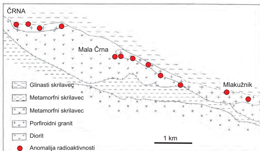
Slika 14: Geološka karta z anomalijami radioaktivnosti jugovzhodno od Črne na Koroškem (prirejeno po Omaljevu, 1971)
