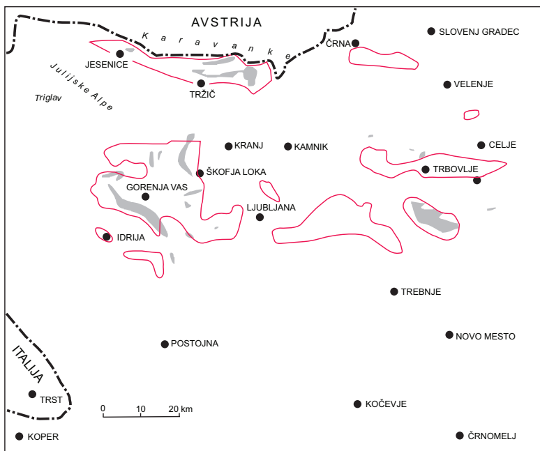
Slika 3: Skica radiometrično raziskanih delov Slovenije (Omajev, 1971)
