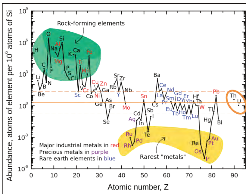
Slika 1: Obilnost kemičnih prvin v Zemljini skorji (v atomih elementa na 10^6 atomov silicija (Si)) (Vir: Internet 4 in 5)
