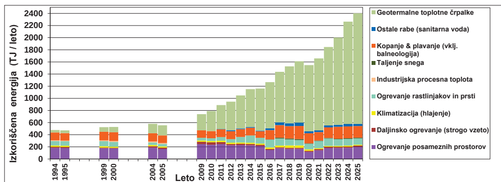
Slika 8: Trendi izkoriščene geotermalne energije po kategorijah neposredne rabe toplote v Sloveniji v obdobju 1994–2025 (skupna izkoriščena energija v letu 2025: 2400,83 Tj)
