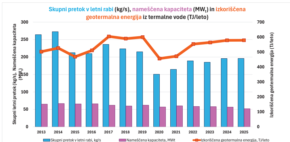
Slika 5: Skupni pretok v dejanski letni rabi ( kg/s ), nameščena kapaciteta vrtin ( MW_t ) in izkoriščena geotermalna energija ( TJ/leto ) do leta 2025
