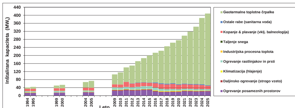
Slika 7: Spremembe inštalirane toplotne moči po kategorijah neposredne rabe toplote iz geotermalne energije v Sloveniji v obdobju 1994–2025 (skupna kapaciteta naprav v 2025: 408,62 MW.)
