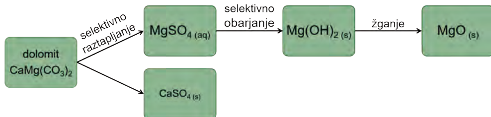
Slika 6: Shema pridobivanja različnih produktov iz dolomita
