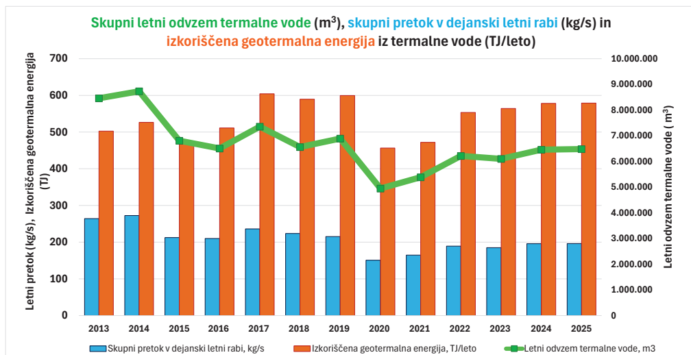
Slika 4: Skupni letni odvzem termalne vode ( m^3 ), pretok v dejanski letni rabi ( kg/s ) in izkoriščena geotermalna energija ( TJ/leto ) do leta 2025 (skupni letni odvzem pred letom 2016 ni povsem zanesljiv).
