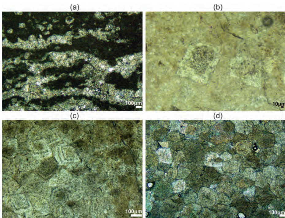
Slika 2: (a) Dolomit s temnimi stromatolitnimi in svetlimi sparitnimi dolomitnimi laminami – Kot pri Ribnici, (b) evhedralni kristali dolomita v kremenčevi (roženčevi) matrici – Kozlov rob, (c) sparitni dolomit z rombičnimi kristali dolomita in rombično osrednjo cono – Hrast pri Vinici, (d) sparitni dolomit s subhedralnimi zrni dolomita.
