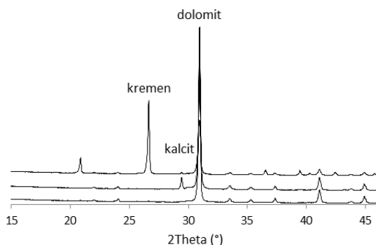
Slika 3: Rentgenogrami izbranih slovenskih zgornjevermskih dolomitov
