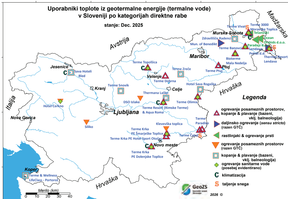
Slika 6: Uporabniki toplote iz GE (termalne vode) v Sloveniji po kategorijah direktne rabe (stanje: 31. dec. 2025); dodan je še daljinski sistem ogrevanja v Benediktu, ki deluje kot zaprti sistem z globoko geosondo in ne izkorišča termalne vode.
