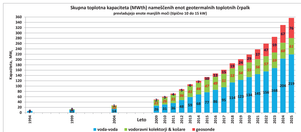
Slika 13: Skupna toplotna kapaciteta (MW) delujočih enot GTČ po vrsti postavitve od začetka vodenja statistike; skupna kapaciteta ob koncu 2025: 356,6 MW t ; za leta 1995–2013 so podatki za kapaciteto (nazivno moč) po vrsti postavitve le približni.
