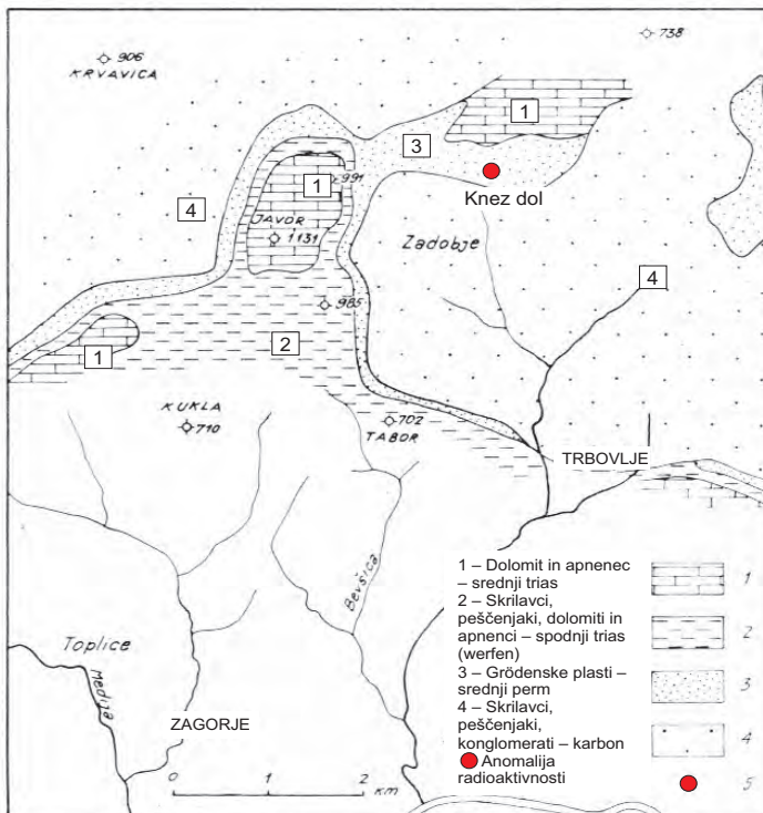
Slika 12: Lokacija Knez dol v grödenskih plasteh (prirejeno po Omaljevu, 1971)
