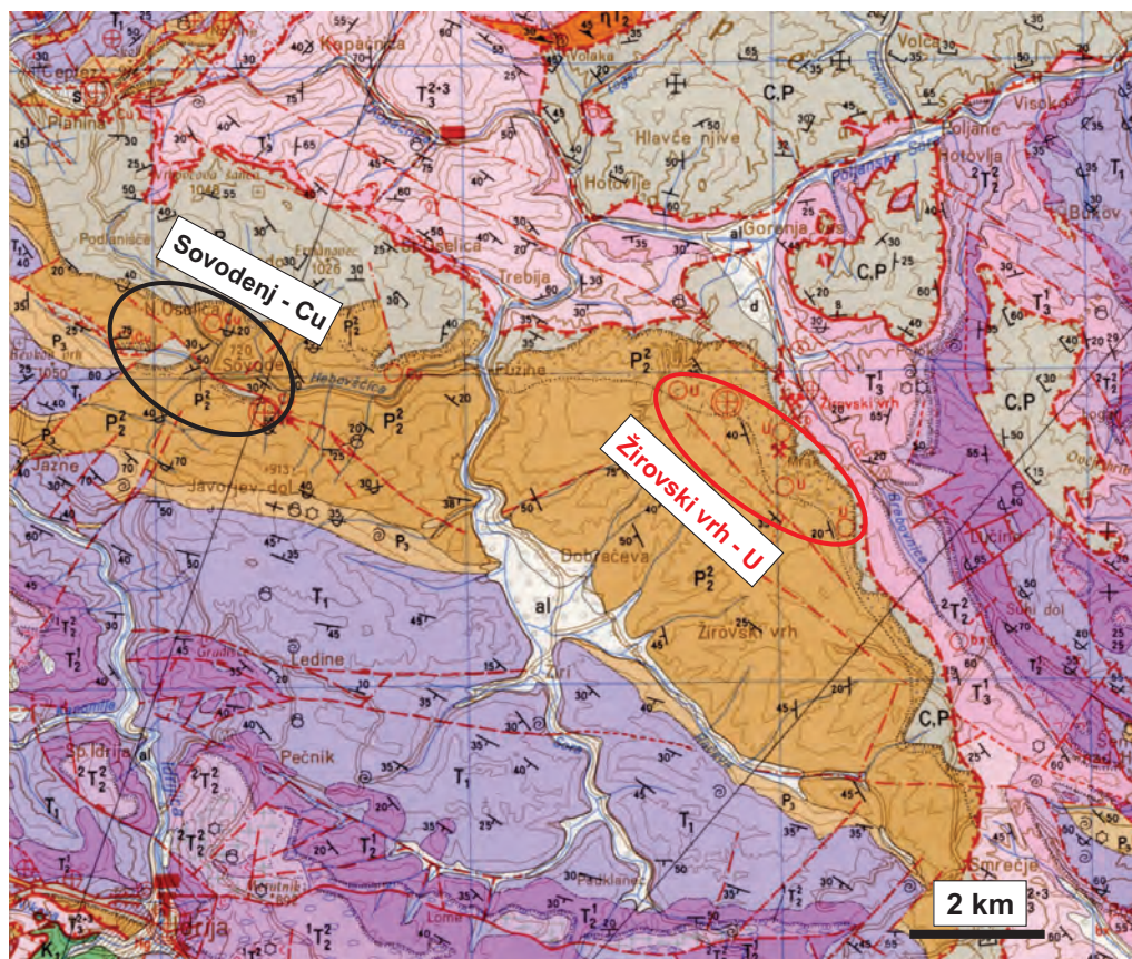
Slika 8: Izsek iz Lista Kranj Osnovne geološke karte (OGK) Jugoslavije 1:100.000 (Grad in Ferjančič, 1974). Grödenske plasti so v rjavi barvi. Prikazani sta območji Žirovski vrh z orudenjem z uranom (U) in Sovodenj z orudenjem z bakrom (Cu).
