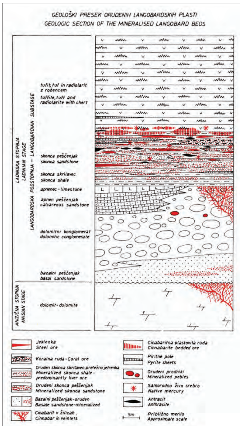
Slika 5: Položaj »skonca« plasti v stolpcu orudenih srednjetriasnih ladinjskih plasti langobardijske podstopnje (Mlakar in Drovenik, 1971)
