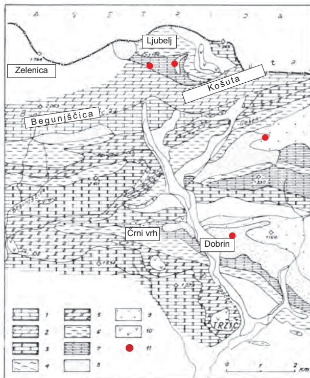
Slika 13: Geološka karta in anomalije radioaktivnosti v Karavankah nad Tržičem (rdeči krožci). Legenda (levo spodaj): 1–6 – triasne plasti; 7 – belerofonski apnenec (zgornji perm); 8 – gródenske plasti; 9–10 – karbonske sedimentne in vulkanogene plasti (prirejeno po Omajevu, 1971).
