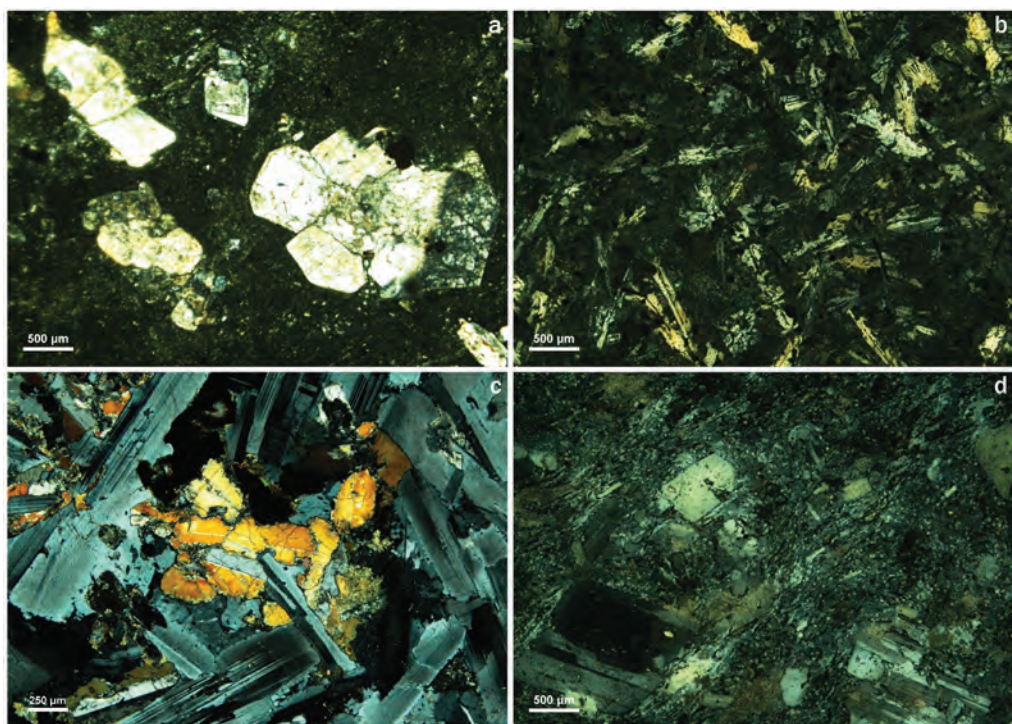
Slika 1: Značilne strukture eruptivnih kamnin. (a) Porfirska struktura: vtrošniki kremena in delno spremenjenih glinenecv v steklasti do kriptokristalni osnovi; pri združevanju vtrošnikov v gručice nastane glomeroporfirska struktura (riolit, Kamna Gorica). (b) Intersertalna struktura: letvice plagioklazov tvorijo ogrodje, vmesne prostore pa zapolnjuje steklasta do kriptokristalna osnova (diabaz, Javorje). (c) Subofitska struktura: vključki paličastih plagioklazov prodirajo v piroksen (rumene interferenčne barve) (gabrodiorit). (d) Trahitska struktura: subparalelno usmerjene letvice majhnih plagioklazov v osnovi obdajajo posamezne večje kristale glinenecv in kremena (dacit, Suhadolnik). Vse slike so posnete s polarizacijskim optičnim mikroskopom pri vklapljenem analizatorju. (Foto: Mirjam Vrabec)
