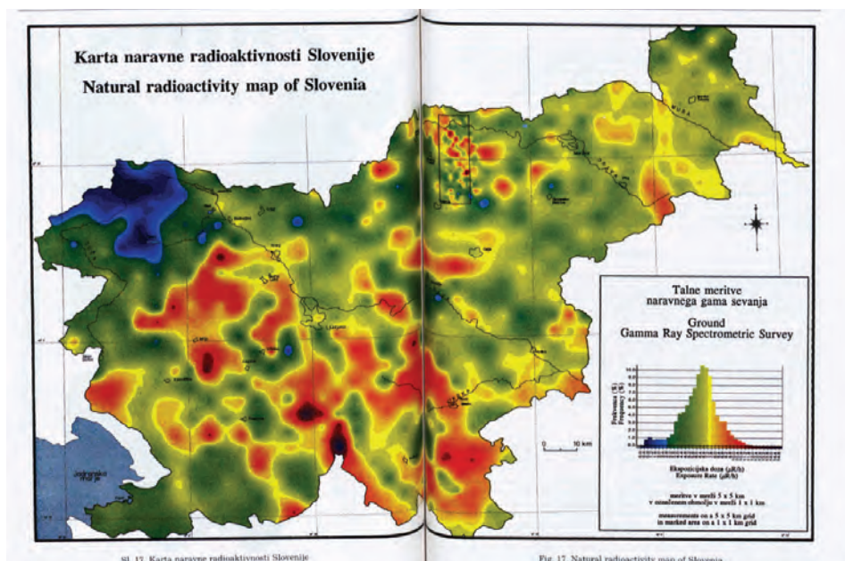
Slika 16: Radiometrična karta tal Slovenije (Andjelov, 1993)
