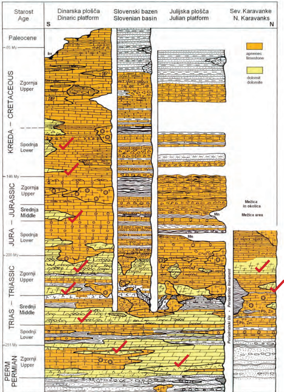
Slika 1: Dolomitne formacije, ki so bile zajete pri vzorčenju. Dopolnjen geološki stolpec je iz članka Ogorelec (2011).
