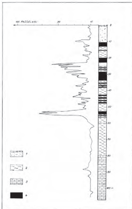
Slika 15: Gama diagram (op.p.: kaže naravno radioaktivnost) vrtnice v rudniku Kočevje (iz: Omaljev, 1971). Legenda (levo spodaj): 1 – preperina; 2 – glina; 3 – apnenec; 4 – premog
