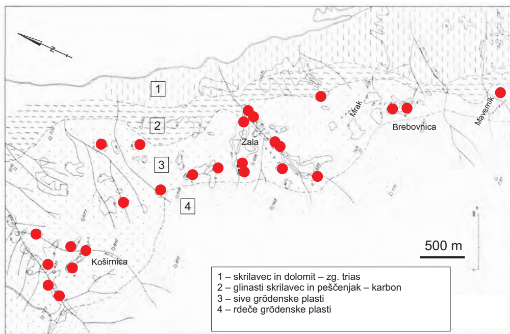
Slika 7: Geološka karta severovzhodnega pobočja Žirovskega vrha s prikazom lokalnosti (rdeči krožci) anomalnih radioaktivnosti nad 100 \mu\text{R/h} (prirejeno po Omaljevu, 1971)
