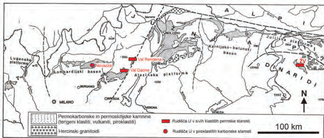
Slika 2: Rudišča urana v Italiji in Žirovski vrh (ŽV) v Sloveniji (Vir: Omaljev, 1982). Rudišče Žirovski vrh je v sivih grödenskih klastitih permske starosti (formacija Val Gardena).
