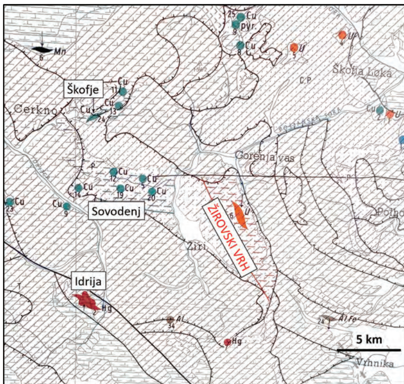
Slika 9: Izsek iz Metalogenetske karte SR Slovenije (Drovenik, F. in soavtorji, 1980), ki kaže območje orudenja z uranom (U) na Žirovskem vrhu, tri pojave U v okolici Škofje Loke, pojave bakra (Cu) na območju Sovodenj in Škofjega ter orudenje z živim srebrom (Hg) na območju Idrije.
