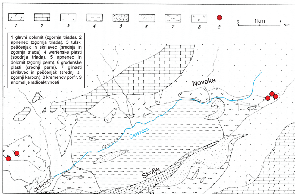
Slika 6: Geološka karta z anomalijami radioaktivnosti (rdeči kroži) v okolici Cerknega (prirejeno po Omaljevu, 1971)
